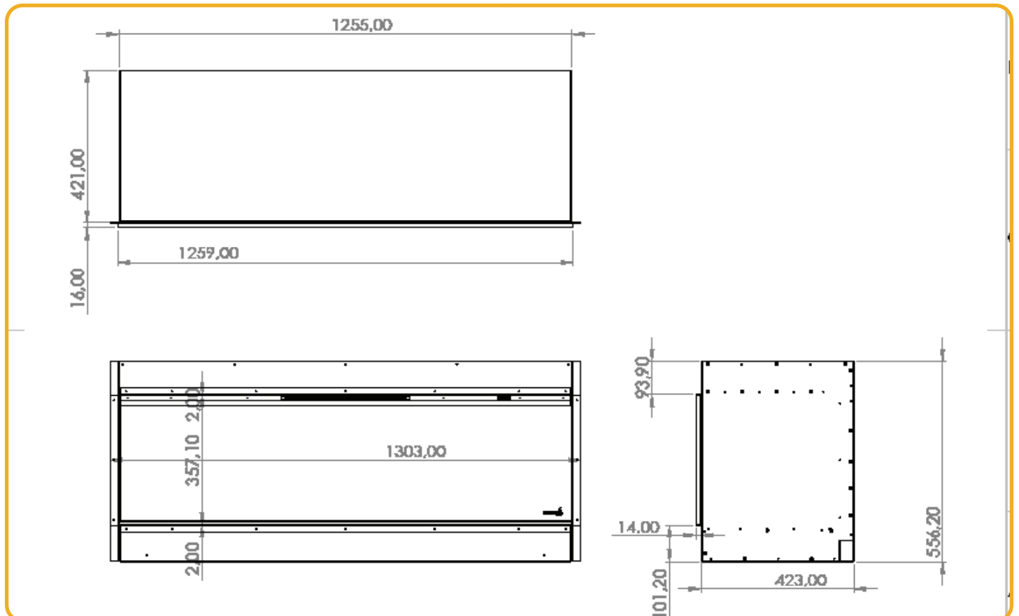
Afb. B.B | Ambiance 125-E F maten
