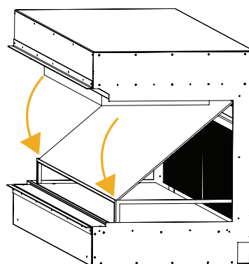
Afb. 9.3 | Zet glas in profiel aan voorzijde
