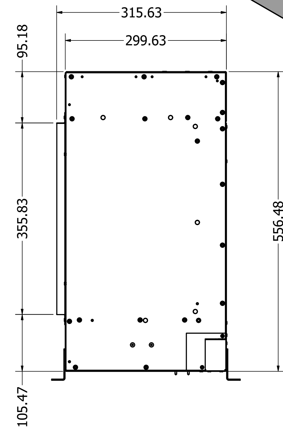
Club 125e Front Alle maten in mm All sizes in mm Alle Größen in mm
