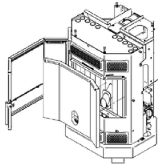
Figuur 2- Vermiculiet brandkamer
