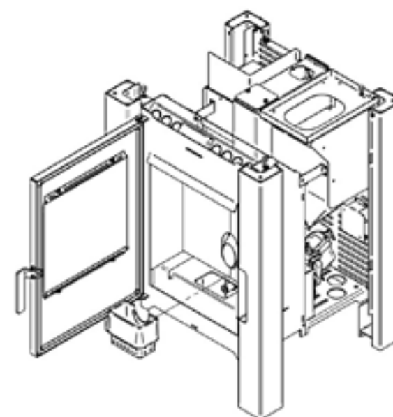
Figuur 1- Brandpot
