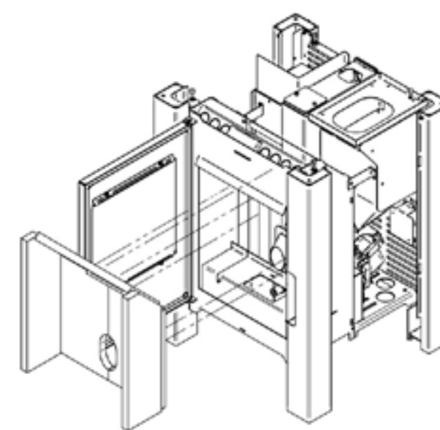
Figuur 2- Vermiculiet brandkamer
