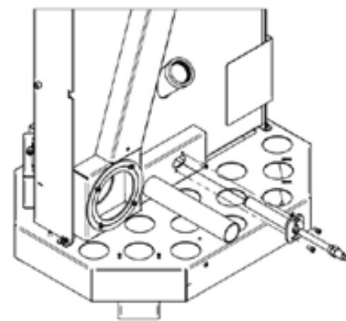
Afbeelding 3- Ontsteker verwijderen
