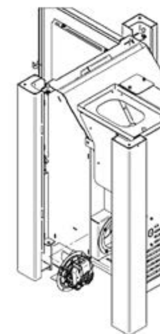
Afbeelding 4- Ventilator verwijderen
