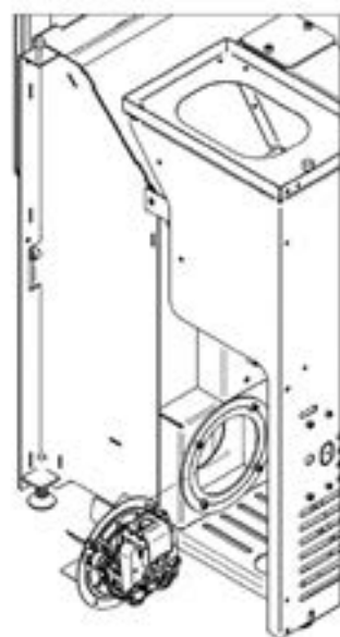
Afbeelding 4- Ventilator verwijderen
