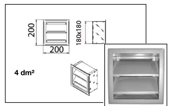
Aanzuigrooster (inlaat)
