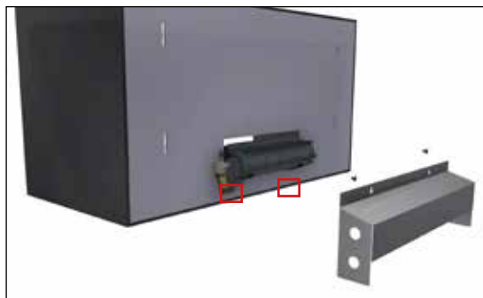
montage beschermkap
