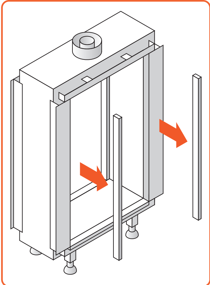
Afb. 10.4 Verwijder zijlijsten
