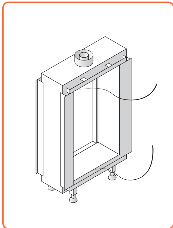
Afb. 10.11 Verwijder glaskkoord
