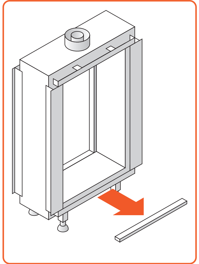
Afb. 10.5 Verwijder onderlijst
