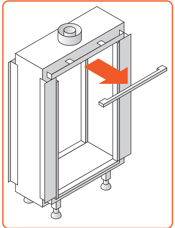
Afb. 10.3 Verwijder bovenlijst
