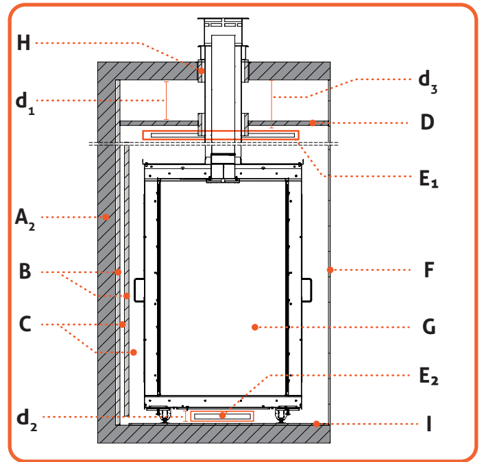
Afb. 6.3 C31: Gas afvoer bij brandbare materialen
