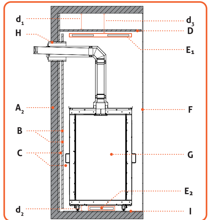
Afb. 6.5 C11: Afvoer bij brandbare materialen
