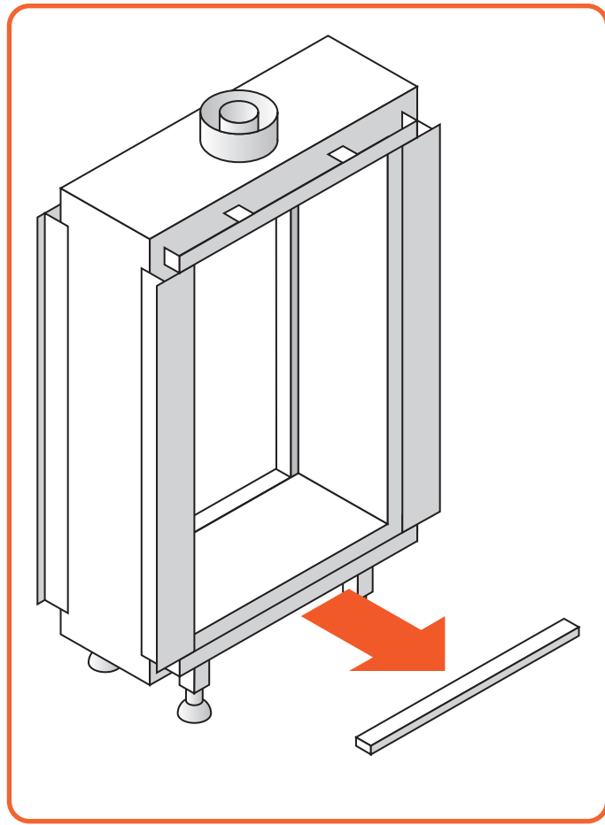
Afb. 9.5 Verwijder onderlijst
