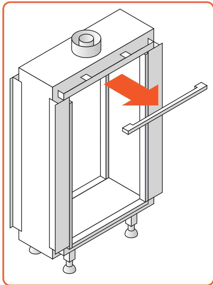
Afb. 9.3 Verwijder bovenlijst
