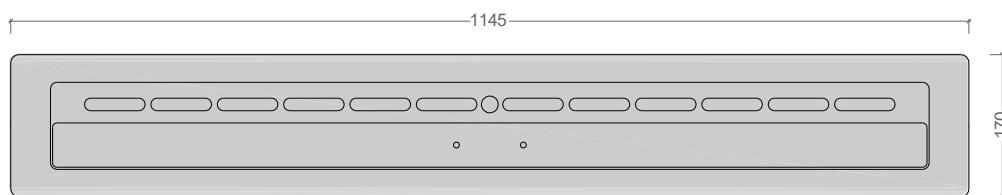
Bovenaanzicht – SB1100
