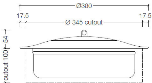
Vooraanzicht
