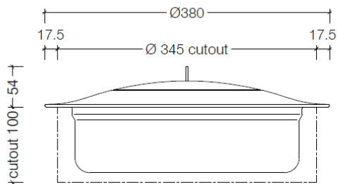
Zijaanzicht
