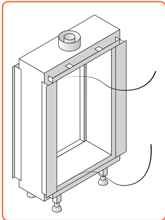
Afb. 10.7 Verwijder glastouw
