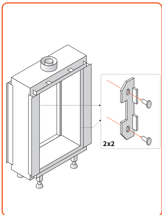
Afb. 10.6 Verwijder glasbeugels
