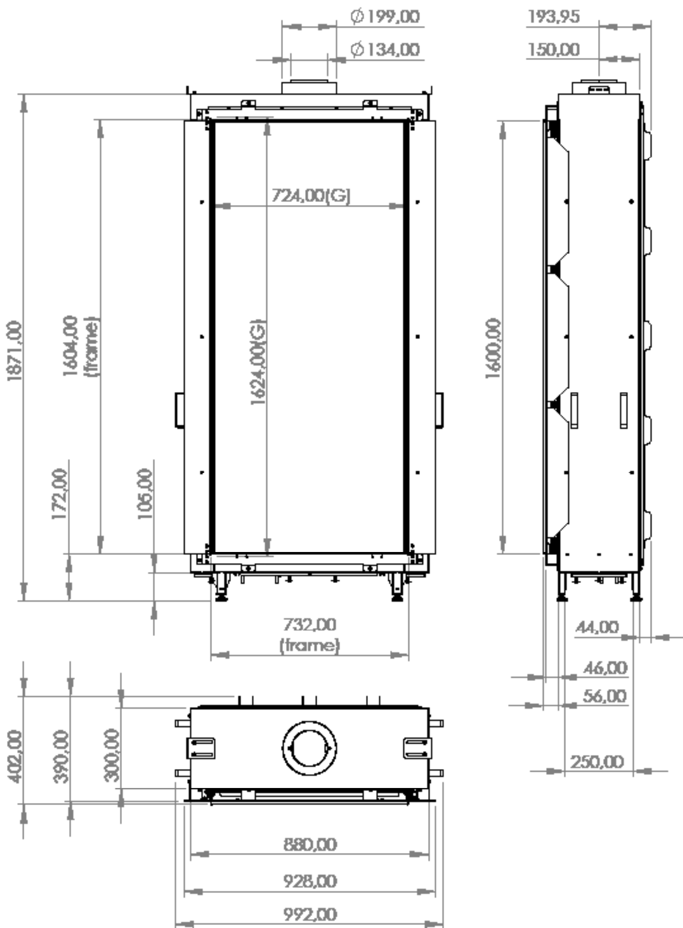
Afbeelding I.A Maattekening van de Sky L F
