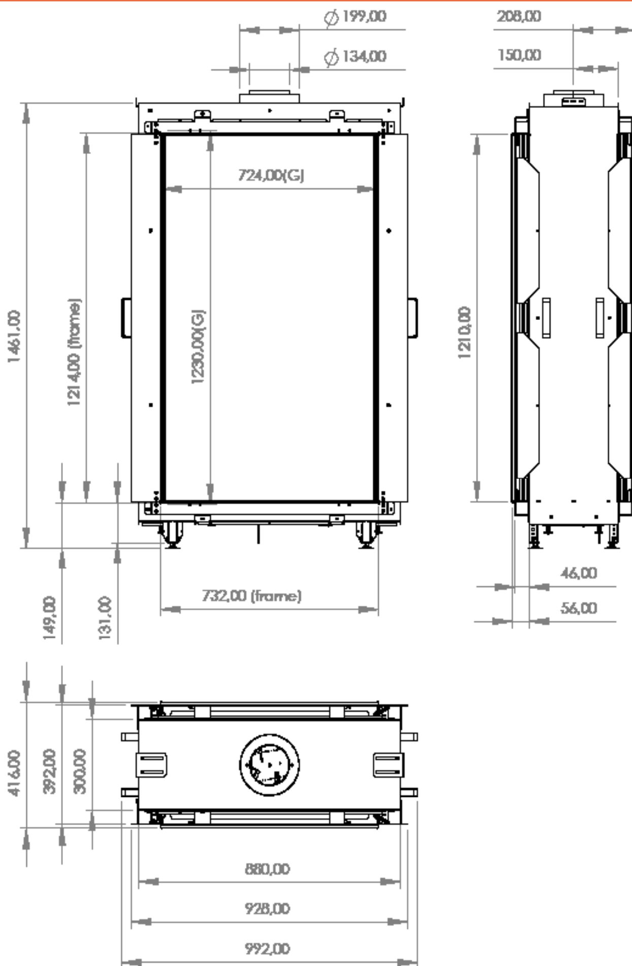
Afbeelding I.A Maattekening van de Sky M T
