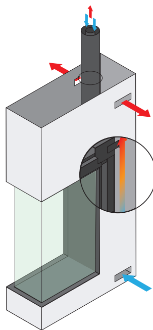
Afb. 5.2 Gebalanceerde aansluiting
